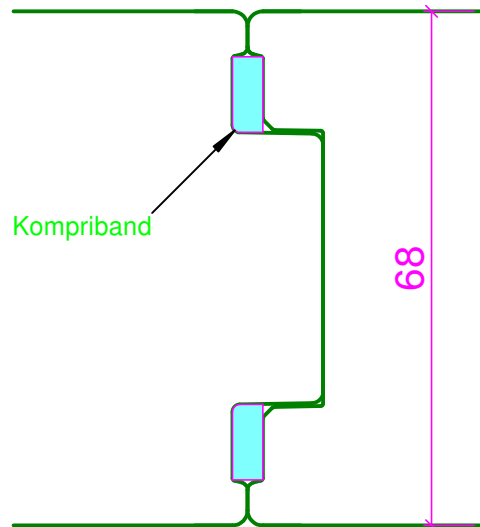
Schnitt A-A Variante 2: mit Koppelnut- und feder
