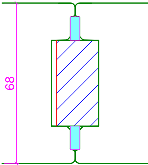
Schnitt A-A Variante 1: mit fremder Feder
