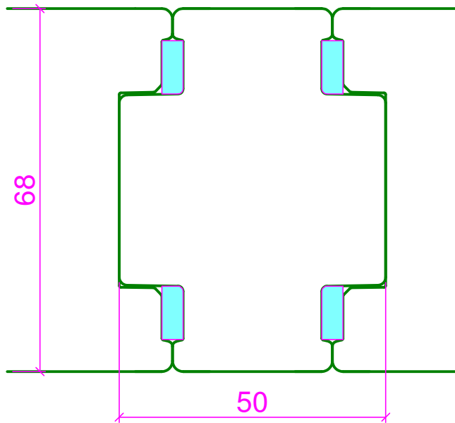
Schnitt A-A Variante 3: mit Koppelleiste
