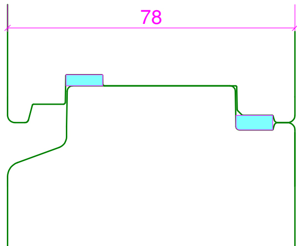
Variante 4: Treppenhauskoppelung
