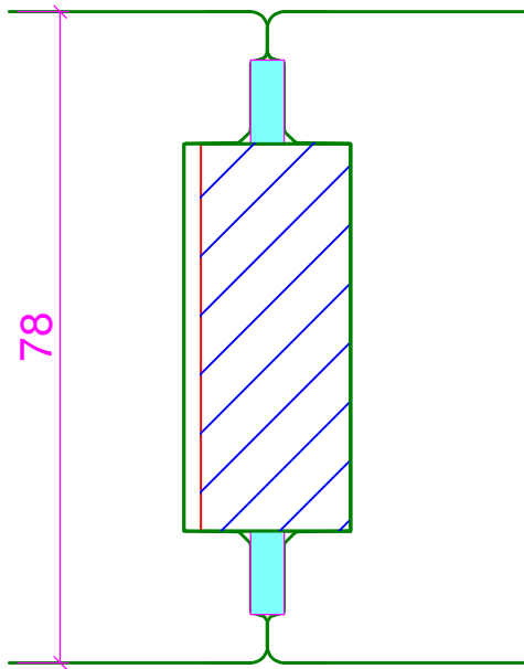
Variante 1: mit fremder Feder
