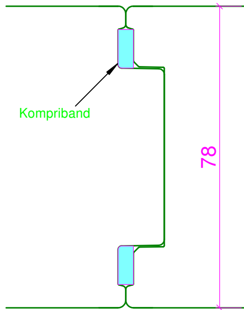
Variante 2: mit Koppelnut- und feder
