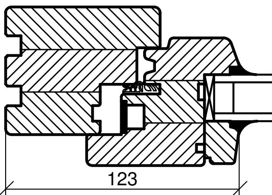
Schnitt C - C
